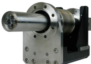
真空4素子シリコンドリフト検出器 XSDD50-04WL ICF114-GP50-Z100 駆動機構付き
