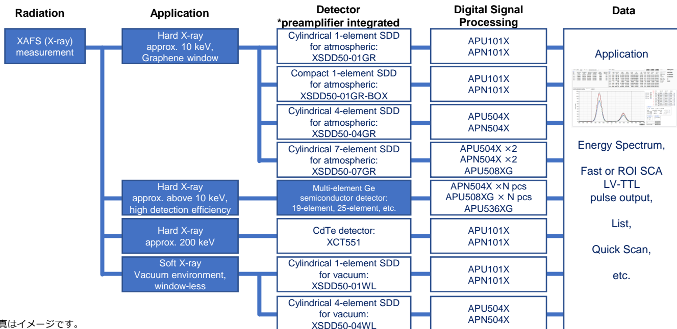
超高計数用ユニット型DSP 36CH APU536XG クイックスキャン1ms, 10Gbps
